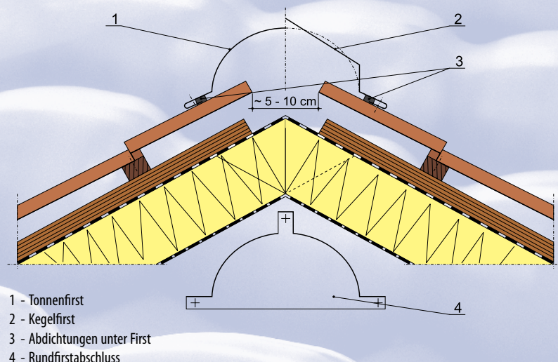
Abb. 13 Beispielmontage des Tonnen- und Kegelfirstes
