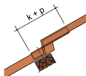
Verbindung der Tafeln am Querfalsz
