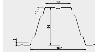
Beispiel für mögliche Perforation T150
